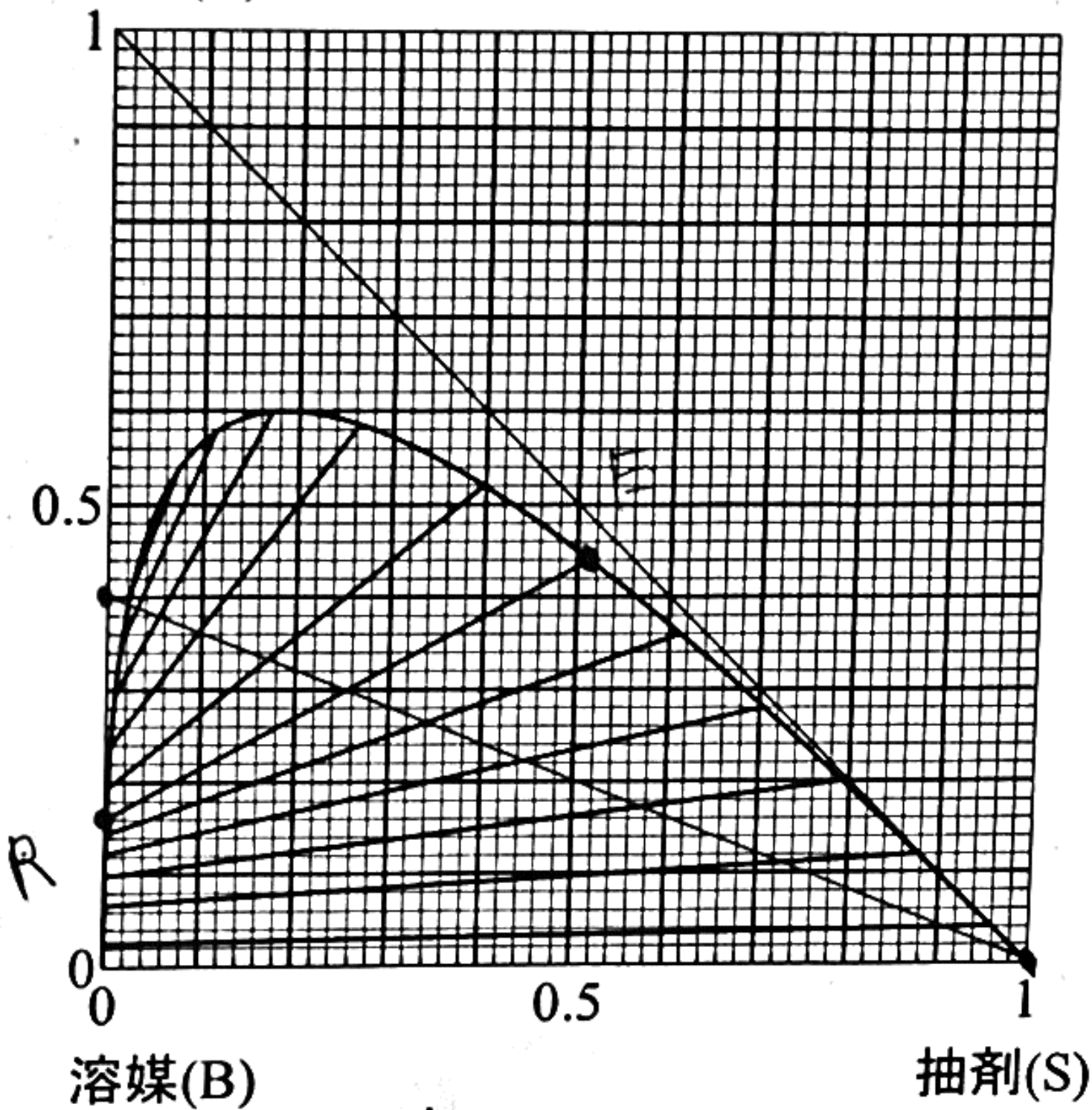
図B? -3 液液平衡関係 (組成はモル分率)
