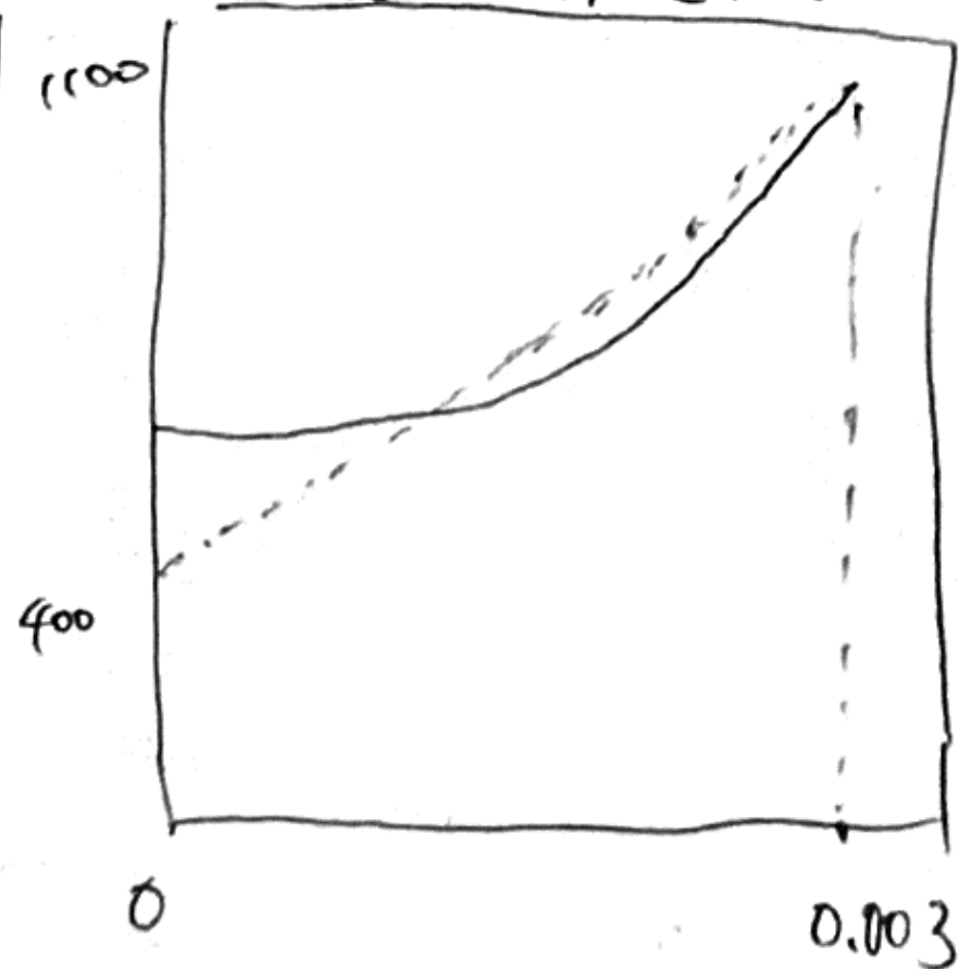
図 B3-4 図 B3-3 の吸収操作に対する \frac{1}{x^* - x} と x のプロット
